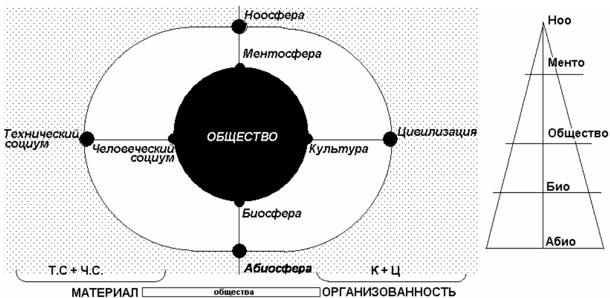
Рис. 8. Место общества в иерархии систем.
